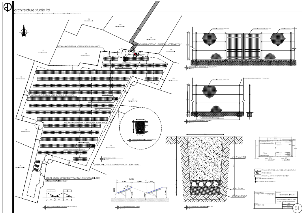
Εικόνα 2.1: Σχεδιασμός προτεινόμενου έργου
