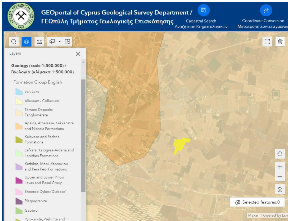
Εικόνα 3.5: Γεωλογικοί σχηματισμοί
